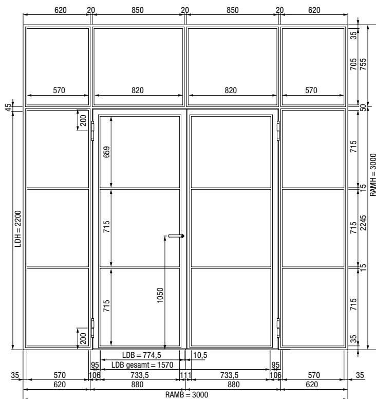
2-flügelige Drehflügeltür mit Seitenteilen und Oberlicht
