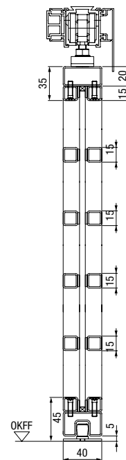
Vertikalschnitt
